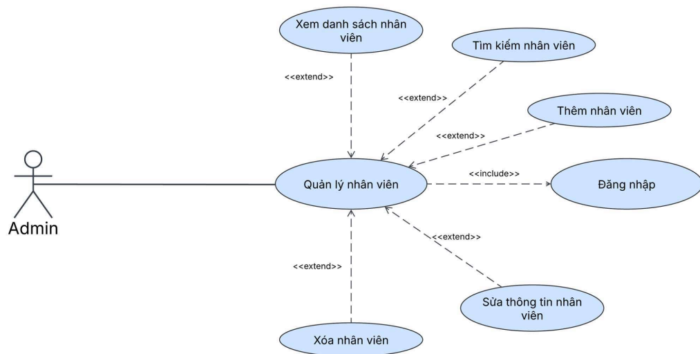
Hình 7 Hình 10: Sơ đồ Use Case Quản lý nhân viên
