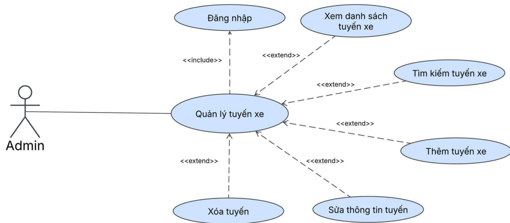
Hình 5: Sơ đồ Use Case Quản lý tuyến xe
