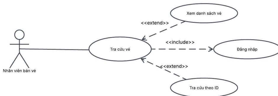
Hình 14: Sơ đồ Use Case Tra cứu vé
