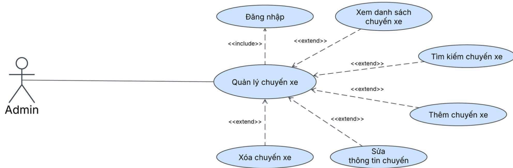
Hình 4: Sơ đồ Use Case Quản lý chuyến xe
