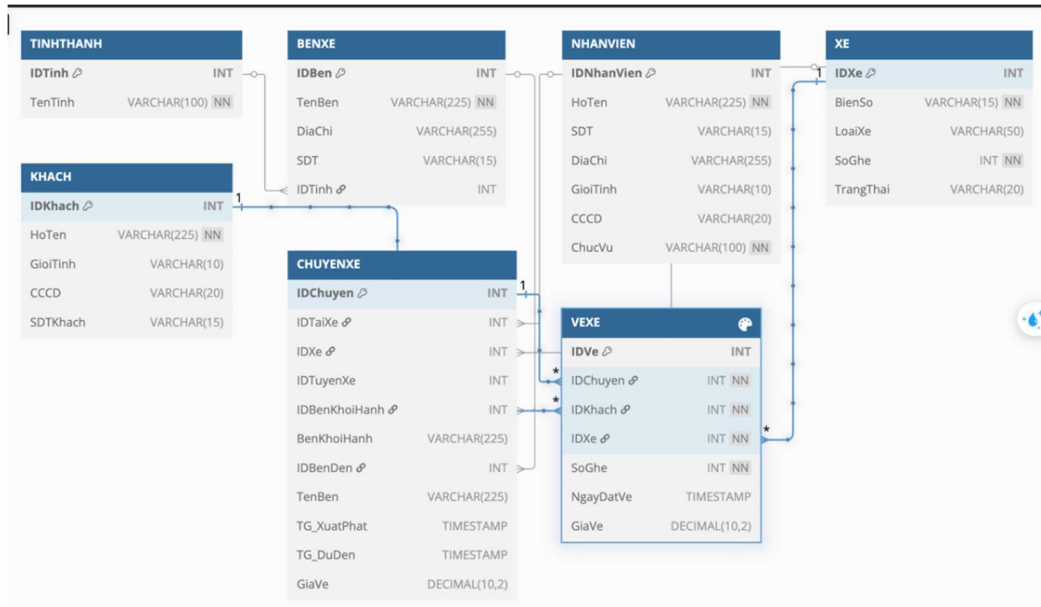
Hình 17: Sơ đồ lớp của hệ thống
